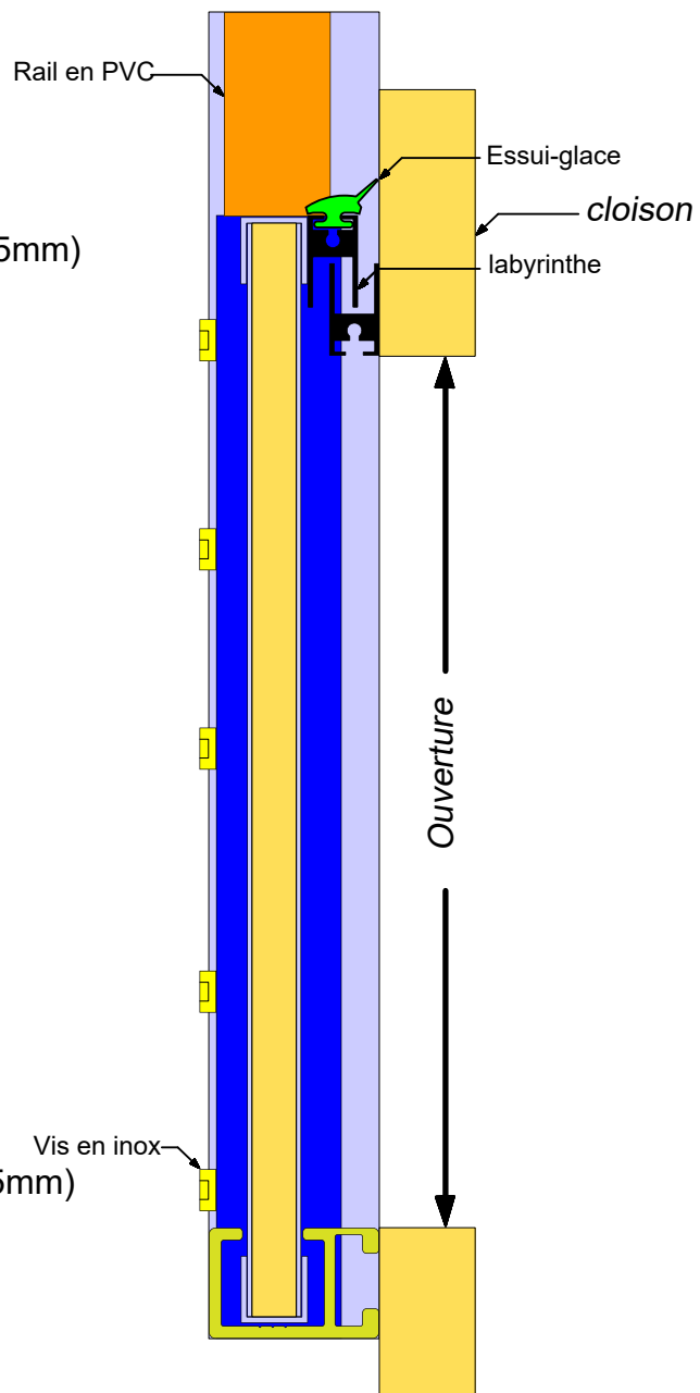
Vue AA
